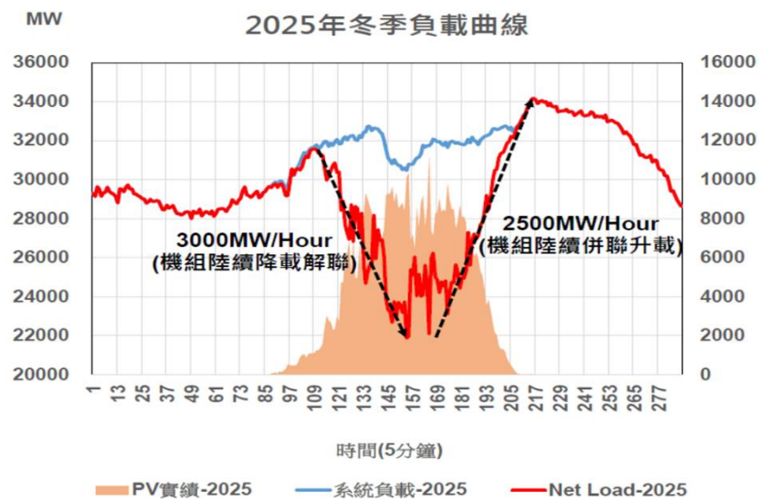
圖 我國2025年冬季之可能用電曲線
